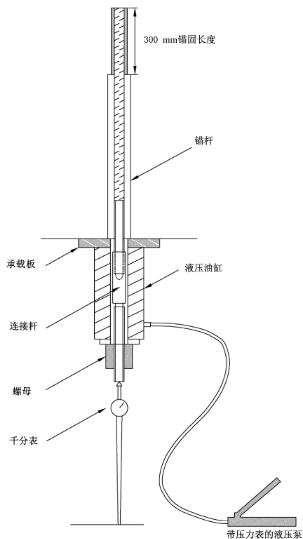
图 A.2 拉拔试验示意图
