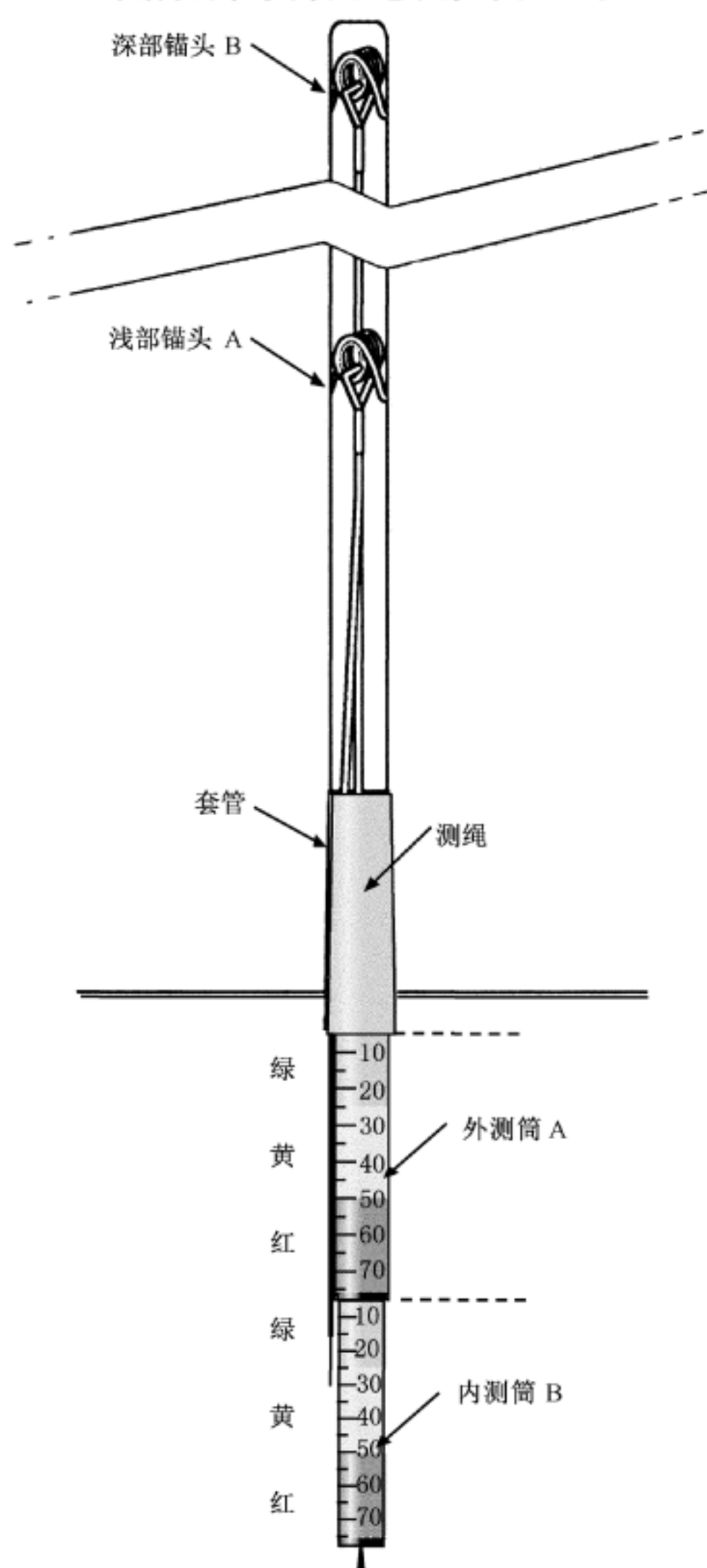
图 C.1 双高度顶板离层指示仪安装示意图
