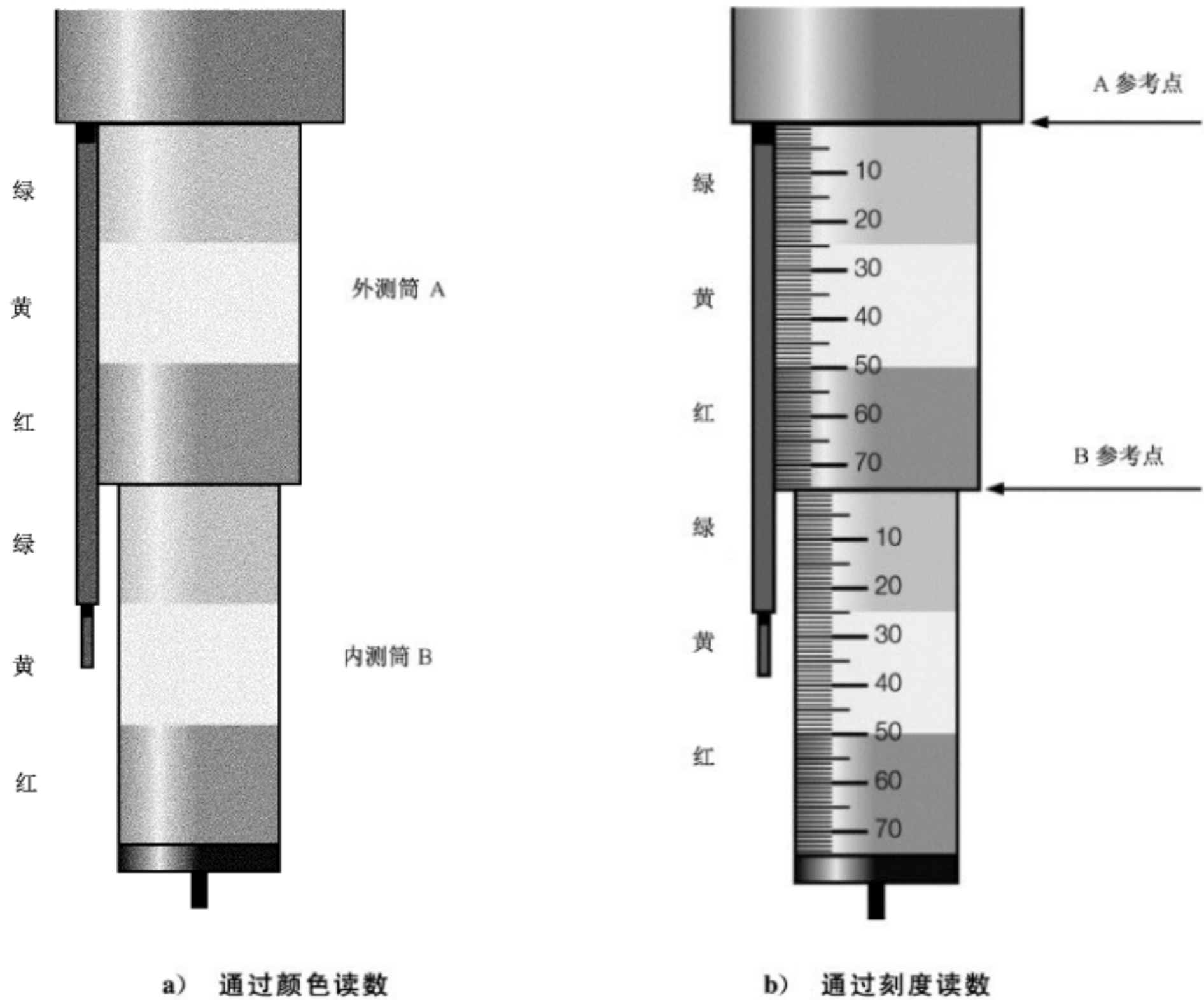
图 C.2 读数方法
